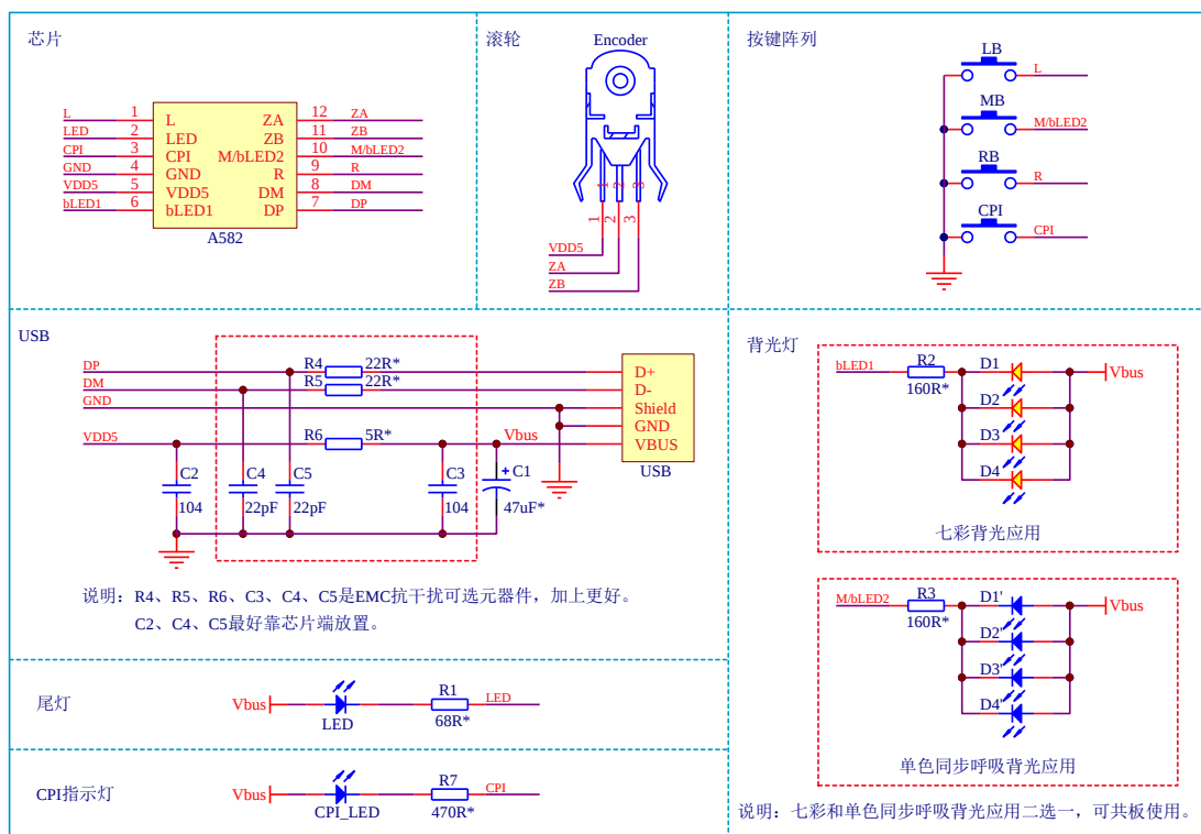
图 3. 应用电路图
