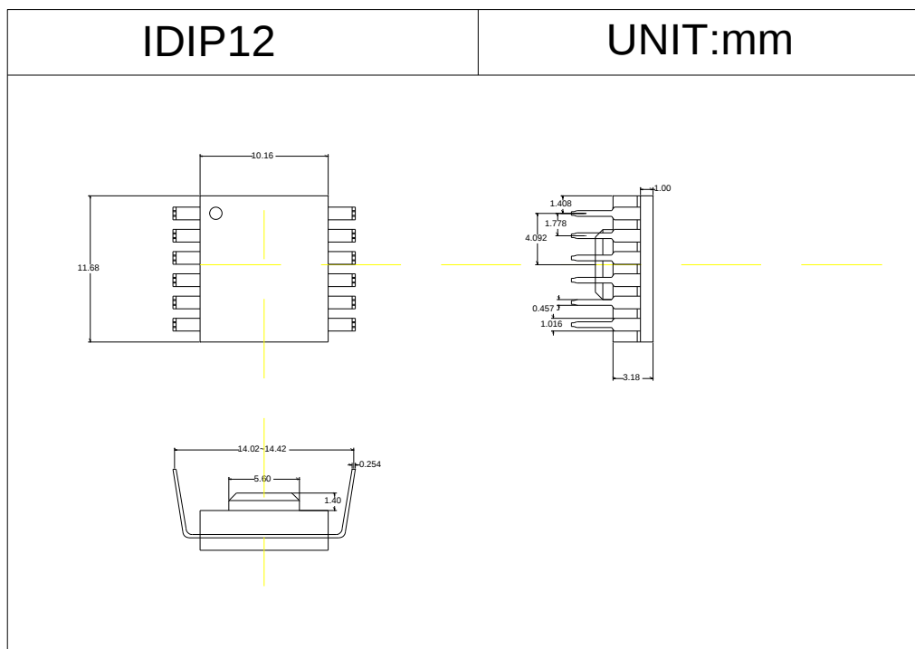
图 4. 封装外观图
