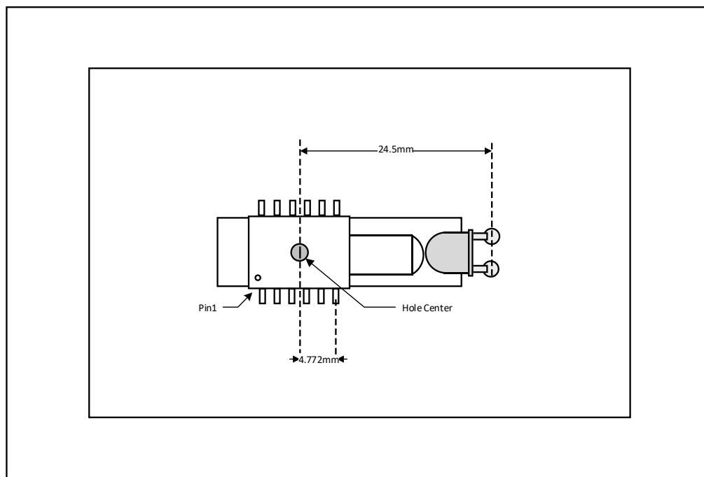
图 5. 2D 装配俯视图
