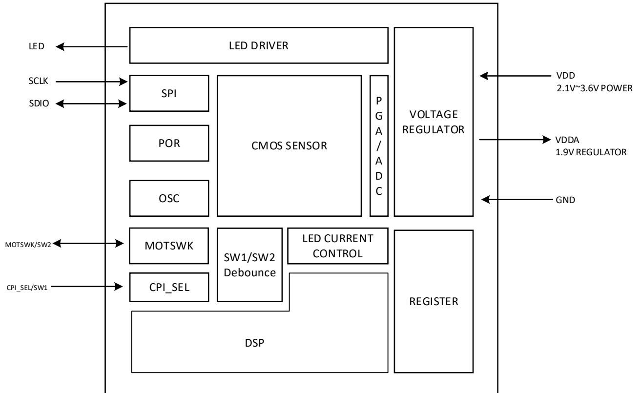
图 3-1 系统框图
