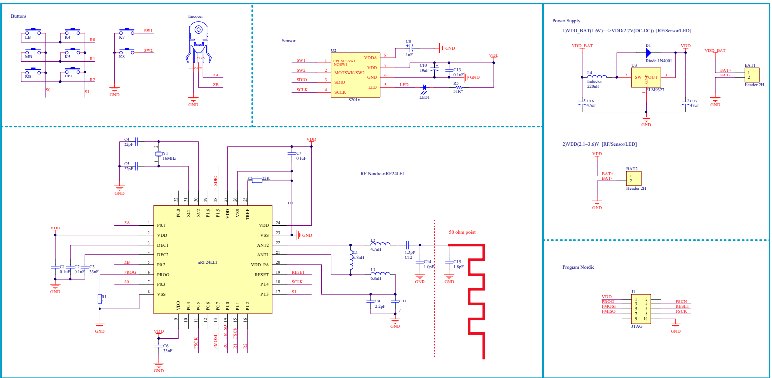
图 11-2 6KEY+2KEY 典型应用电路
