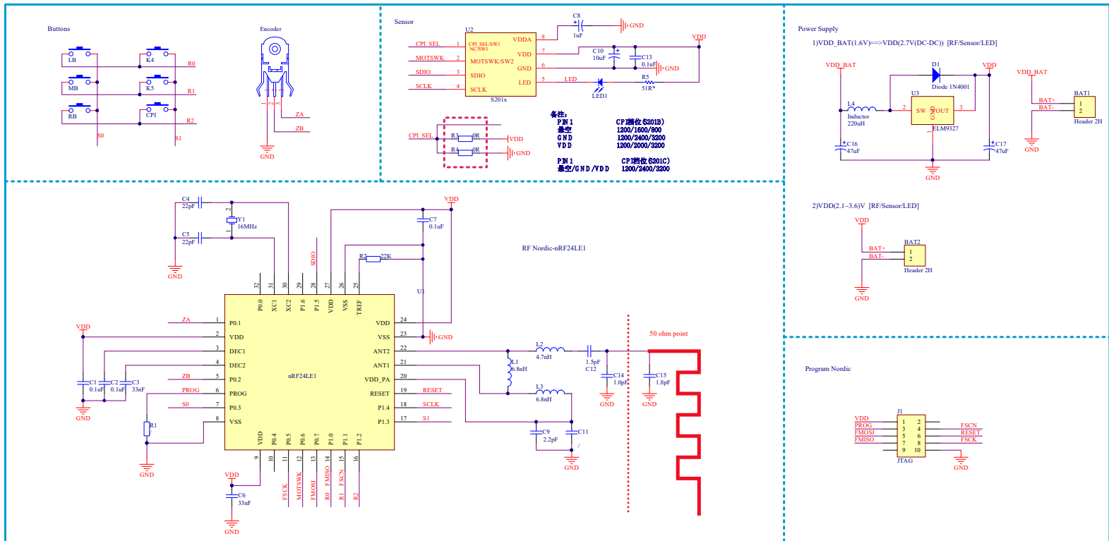
图 11-1 6KEY+CPI_SEL 典型应用电路
